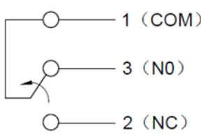
图2 接线示意图
