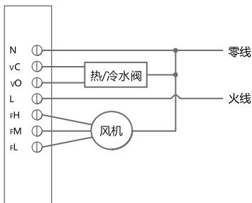
接线图1
